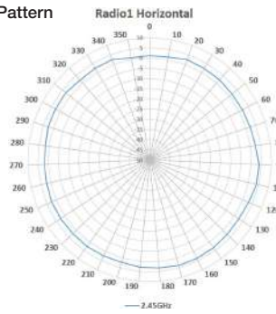
H-Plane Pattern
